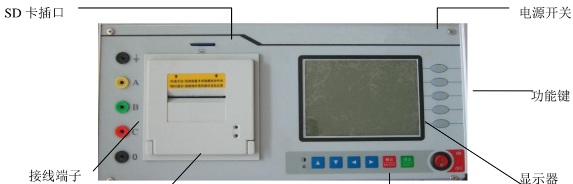
图 1 仪器面板示意图
