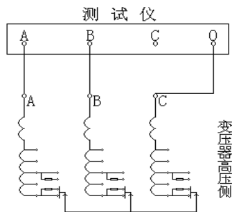
图 21 两相接线图
